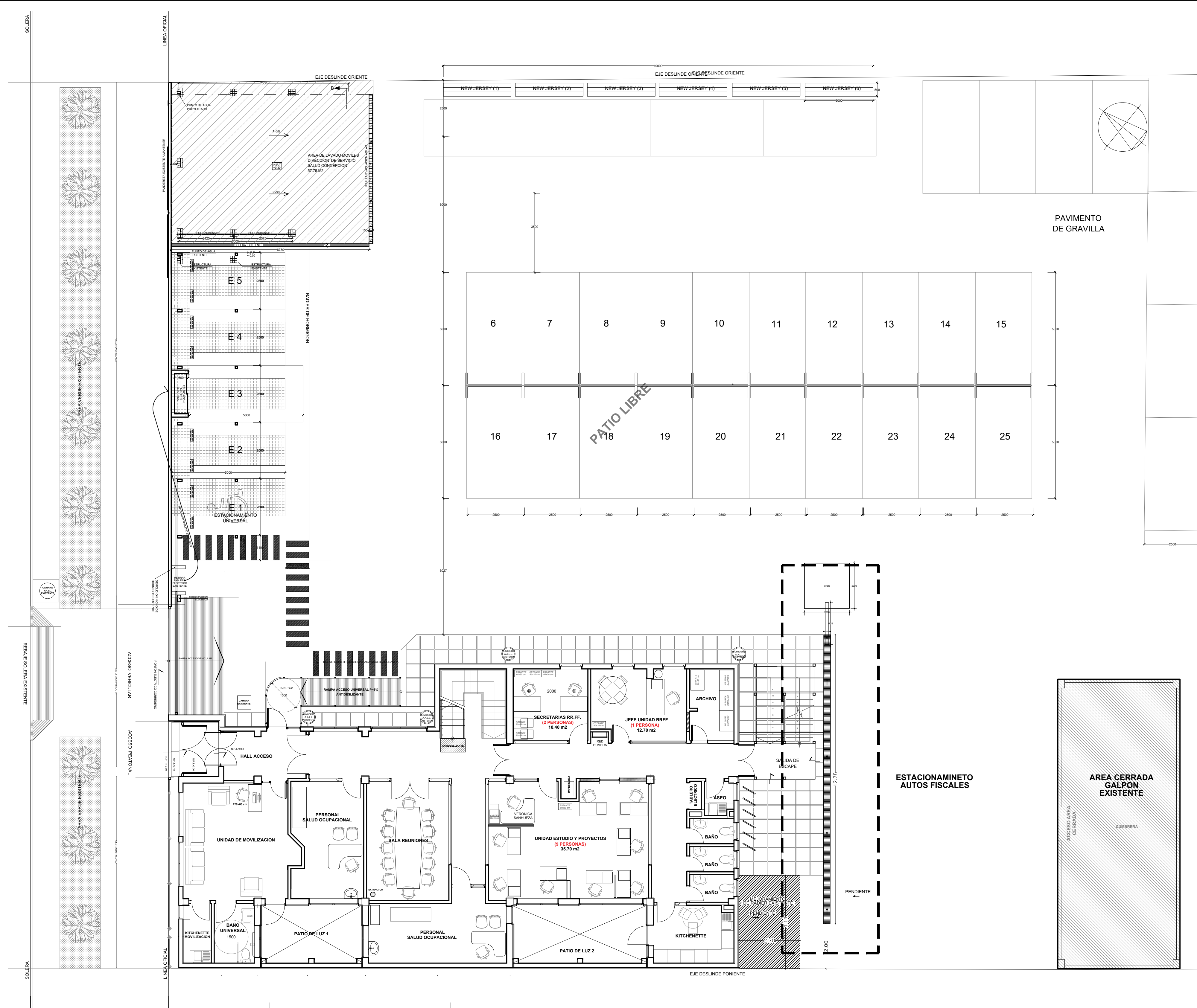
PLANTA DE ARQUITECTURA ESC 1/100
